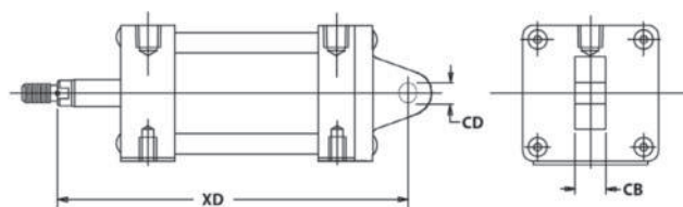
Pivot Model PE
