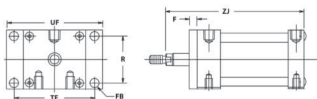
Rod End Flange Model FH*
