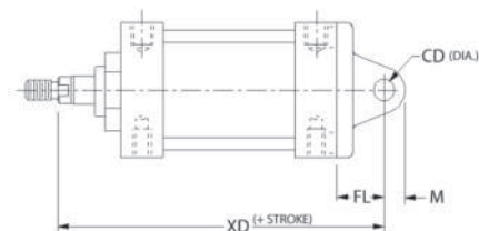
Pivot (PE)
