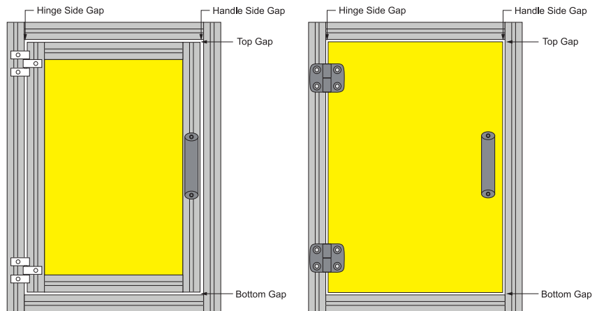
Framed Door
